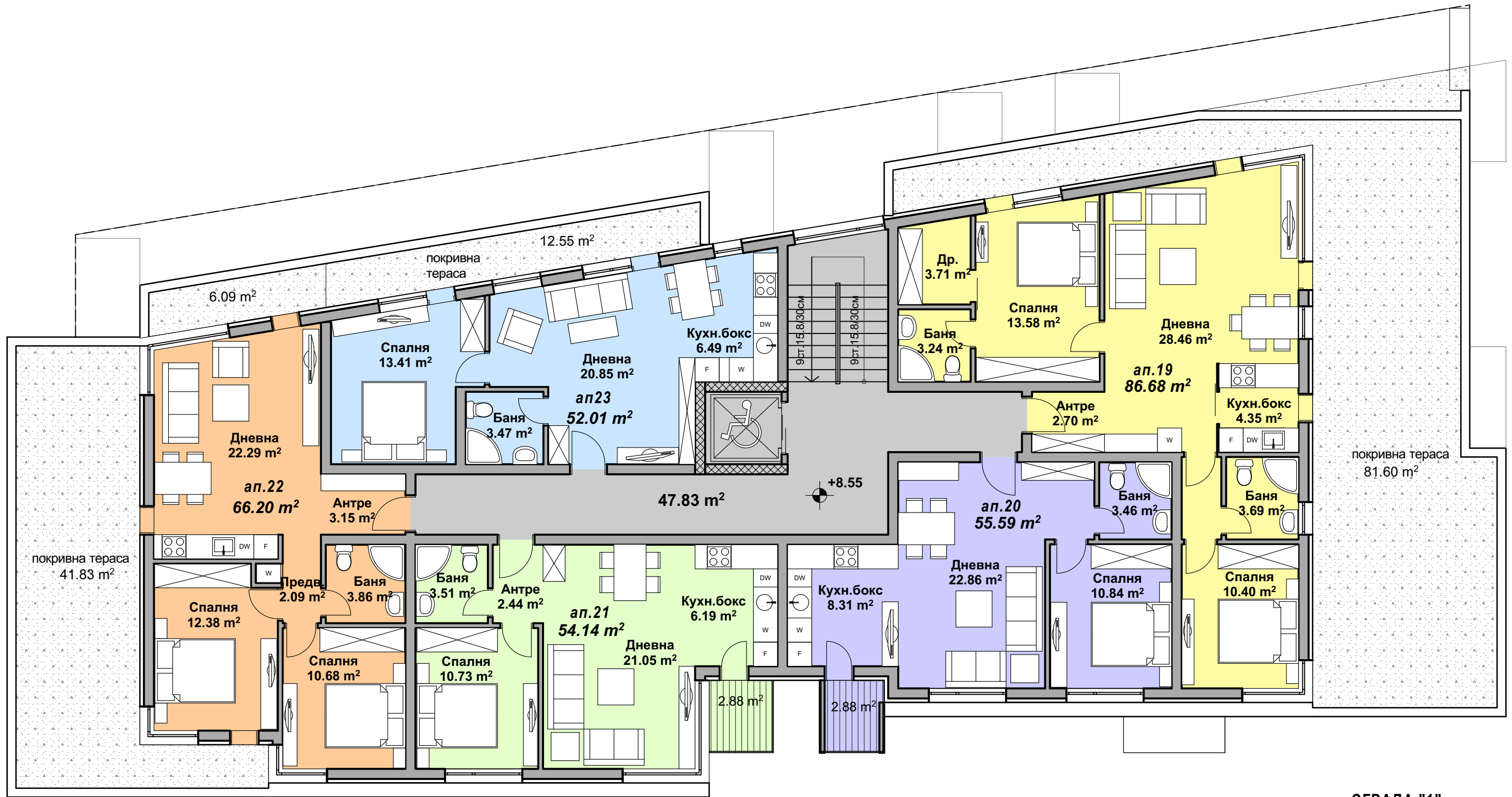
СГРАДА "1" подпокривен етаж: 362.44 m 2
